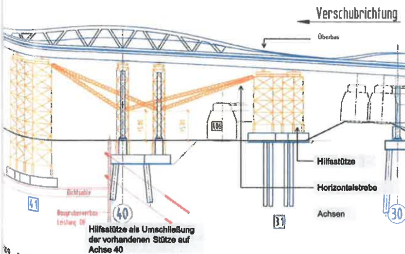
19 Stabilisierungskonzept in der Basisplanung © SEH Engineering GmbH
