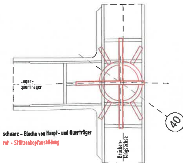
24 Blechanordnung: Ausschottung von Hauptträger (schwarz) und Stützenkopf (rot) © SEH Engineering GmbH
