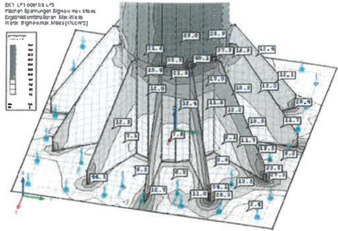
26 Finite-Elemente-Modell des Stützenfußes: Vergleichsspannungen © SEH Engineering GmbH
