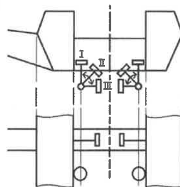
18 Horizontalführung als temporär aktivierbares Drehelement © SEH Engineering GmbH
