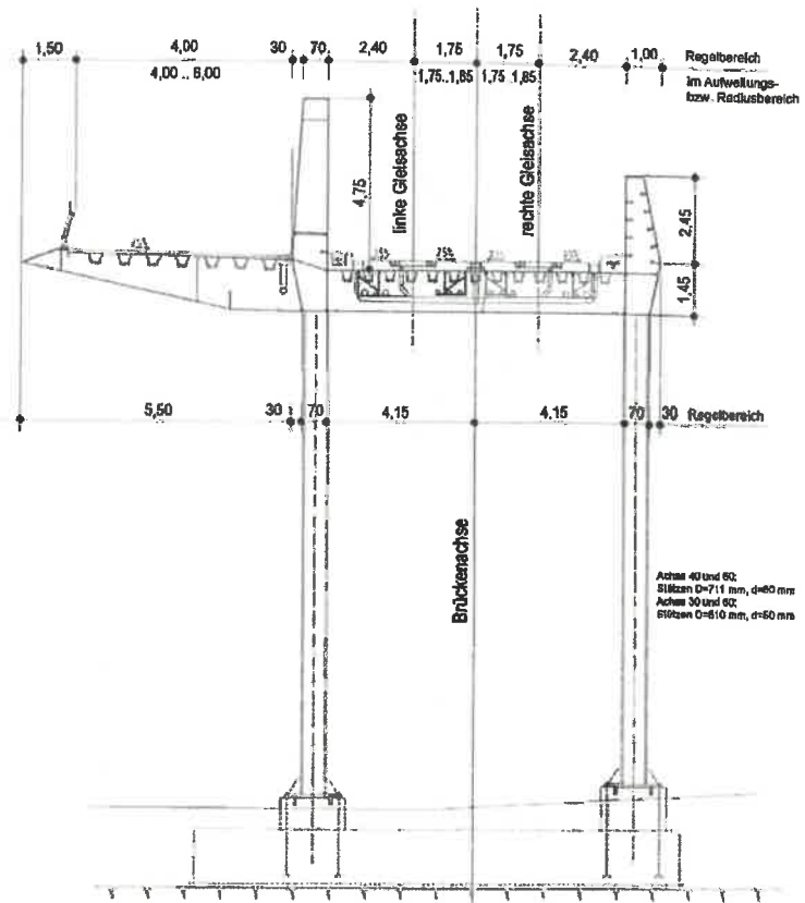
3 Querschnitt im Stützenbereich (Achse 50) © SEH Engineering GmbH
