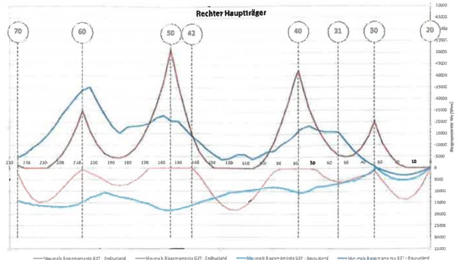
23 Biegemomentenverteilung Endzustand und Bauzustände, rechter Hauptträger © SEH Engineering GmbH
