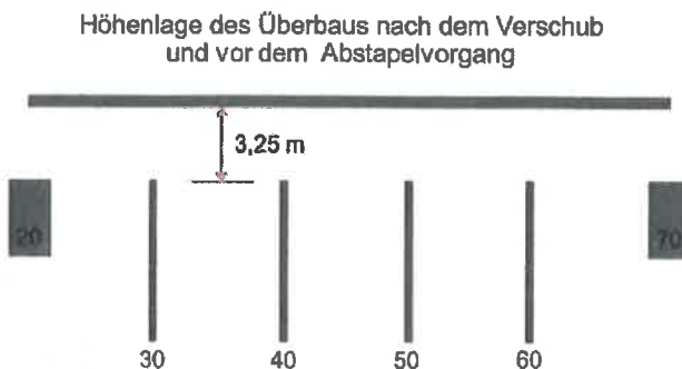
22 Prinzipdarstellung der Abstapelsituation © SEH Engineering GmbH
