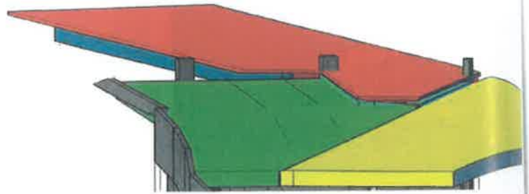
13 Montagebereich aus drei Ebenen: Rampe neu (grün), Rampe Bestand (gelb), temporäre Ebene (rot) © SEH Engineering GmbH
